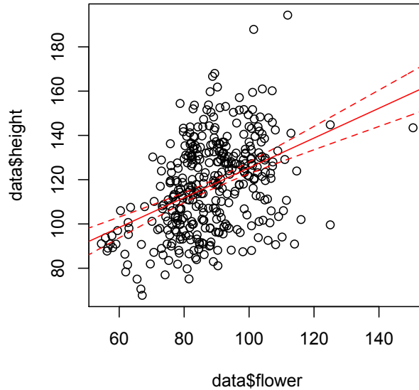
図 8. モデルをあてはめたときの y の信頼区間 x の平均付近は狭く、そこから離れるほど広くなる
