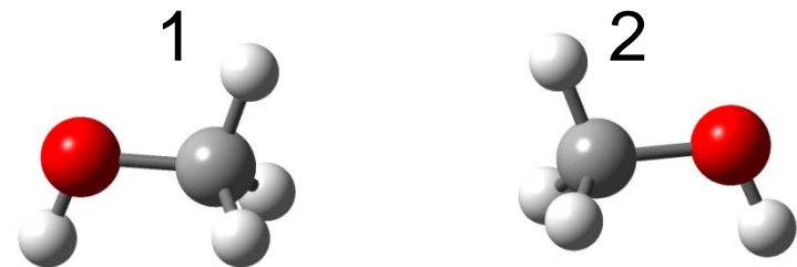
凝縮相
