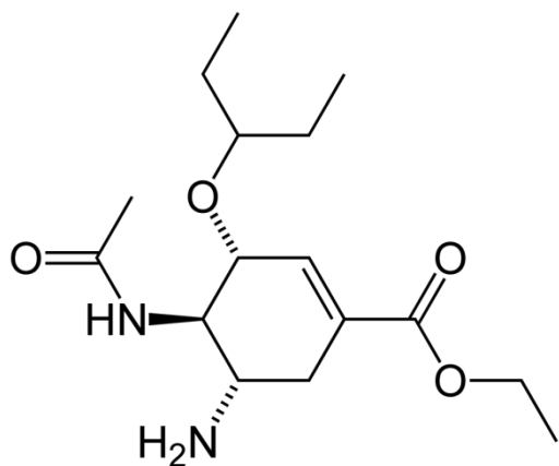
Oseltamivir: インフルエンザ治療薬 (商品名: Tamiflu) 化学式: C_{16}H_{28}N_2O_4
