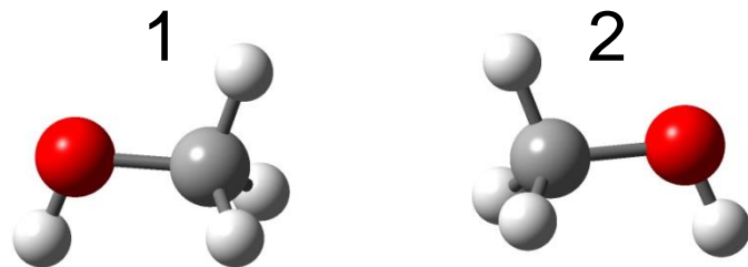
気相
