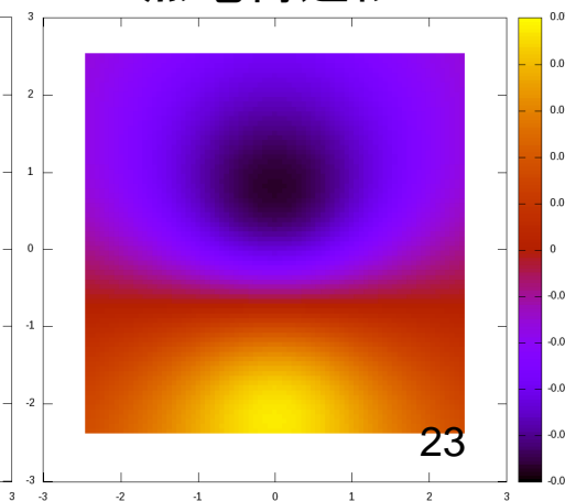
点電荷近似
