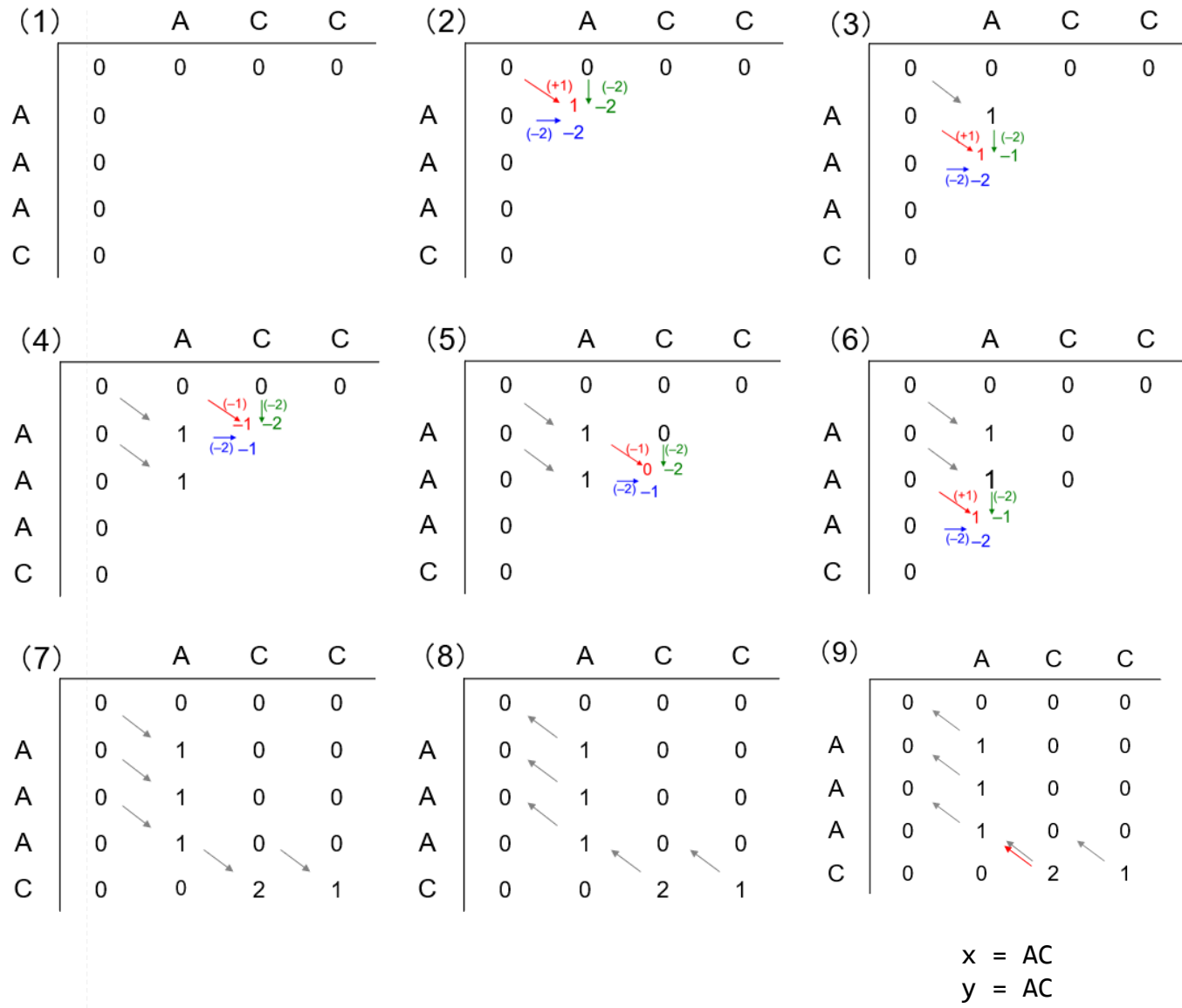
図3.2 最適局所アラインメントの計算例
