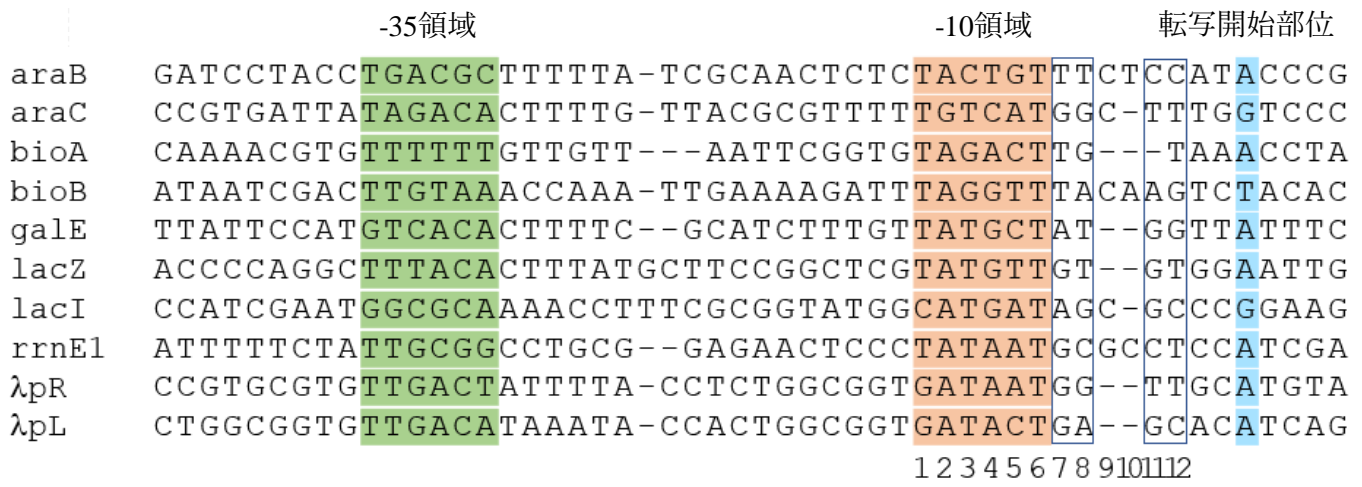
図3.20 プロモータ領域のMSAの例
