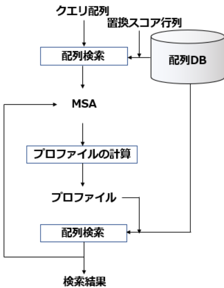
図3.25 PSI-BLASTの処理手順
