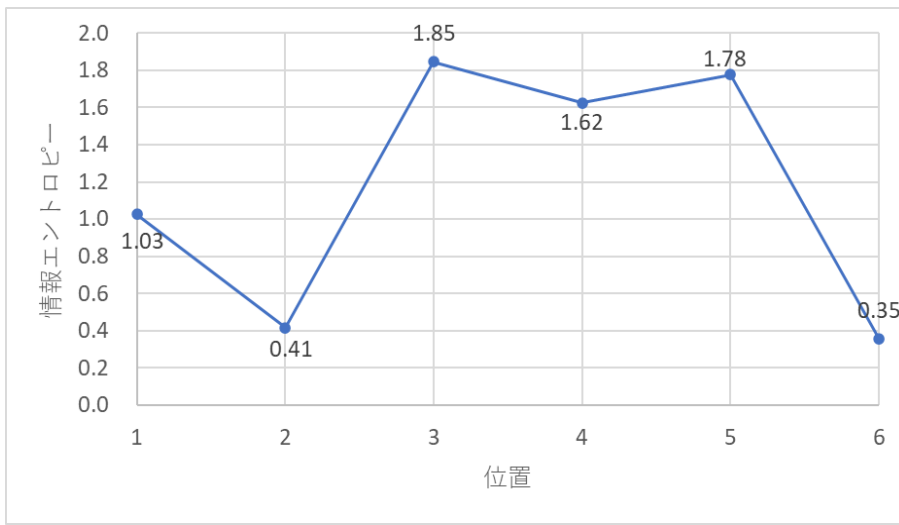
図3.31 プリブノーボックスの情報エントロピーのプロット
