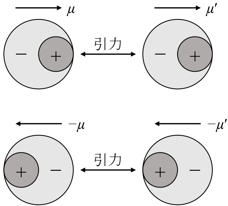
図4.10 van der Waals引力の起源
