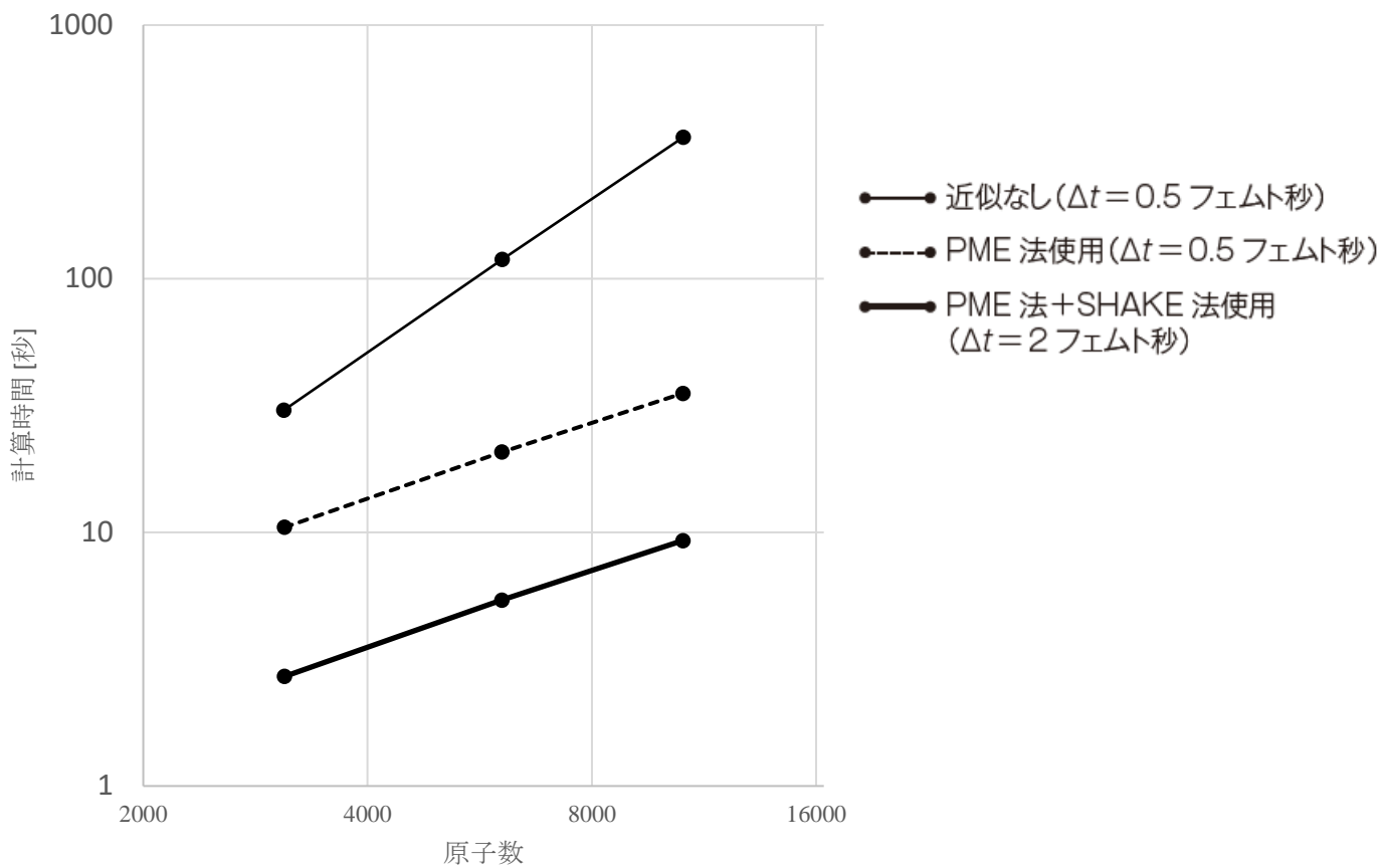
図4.18 分子動力学シミュレーションの計算時間の原子数依存性
