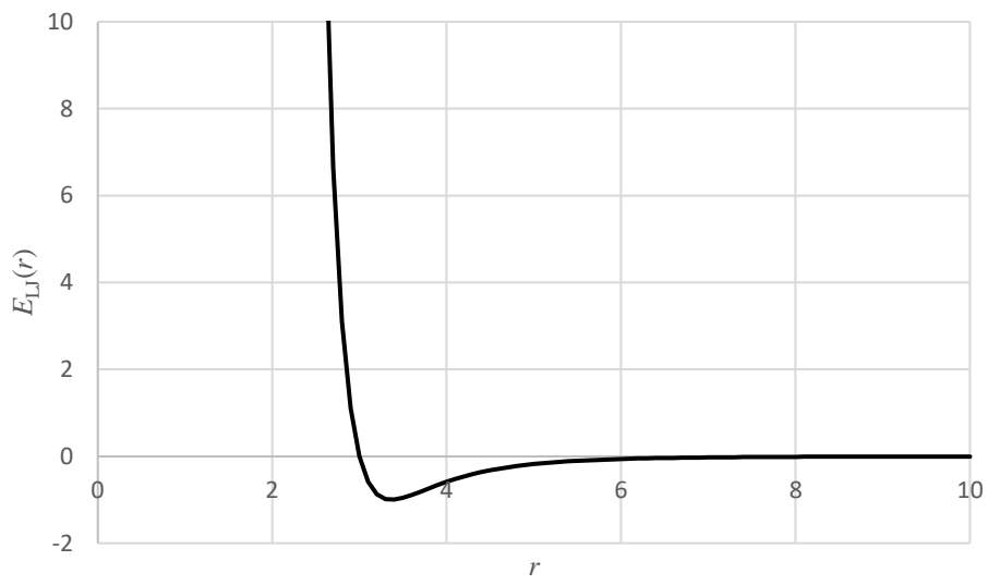
図4.9 Lennard-Jonesポテンシャルの概形 \sigma = 3 、 \varepsilon = 1 とした。
