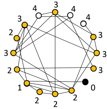
図5.20 (a)規則性のある格子ネットワーク（三角格子）、(b)同じ頂点数のランダムネットワーク 数字は0の頂点を起点とした最短のステップ数。
