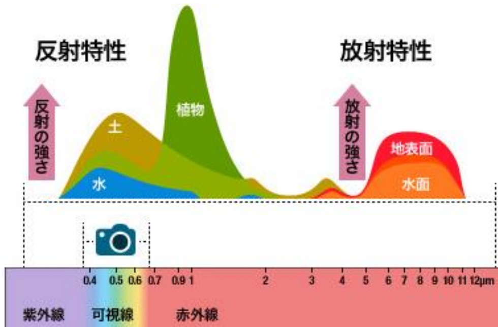
図7.2 植物、土壌、水面などにおける光の反射率の違い 「(c) JAXA 一部改変」
